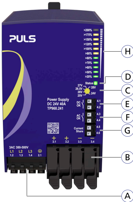
Fig. 18-1: Front side
