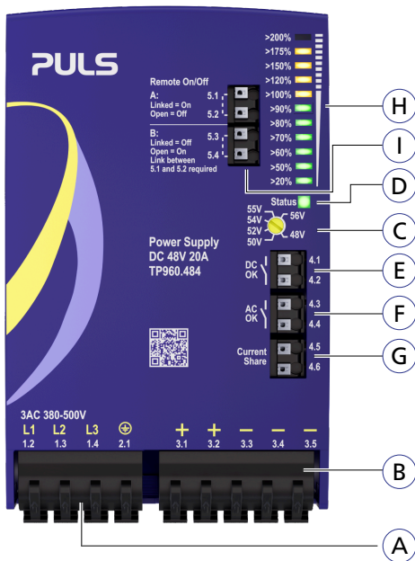
Fig. 19-1: Front side
