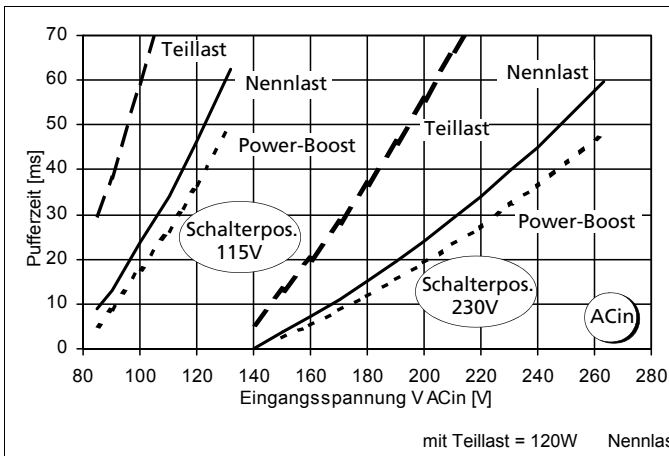
Pufferzeit (typ., bei Vout=24V)
