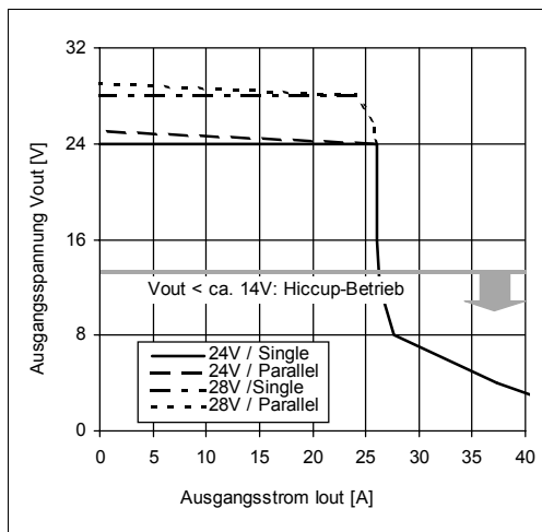
Ausgangskennlinie (typ.)
