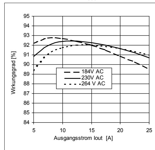
Wirkungsgrad (typ., bei V_{out}=24V )
