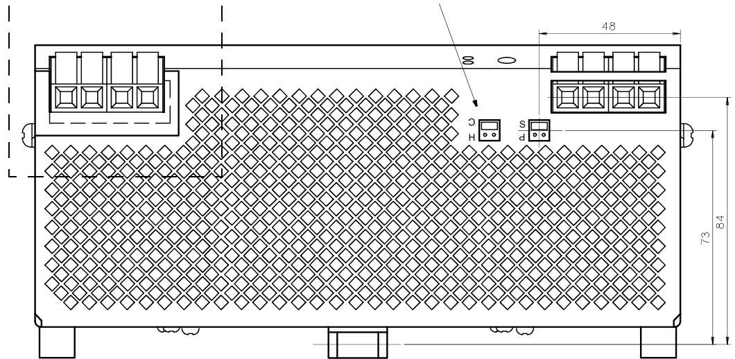
Ansicht SL20 von unten
