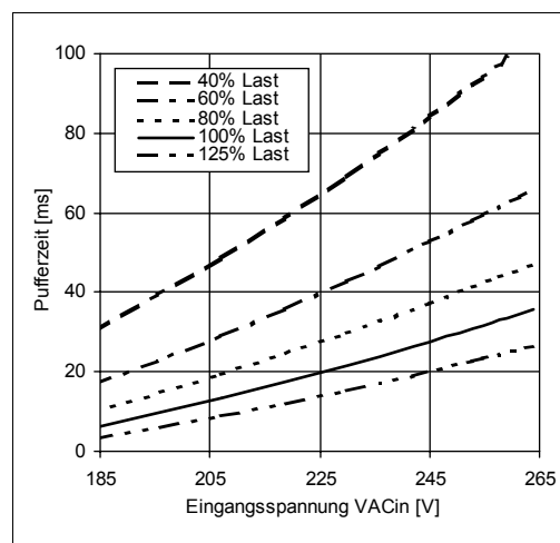
Pufferzeit (min., bei V_{out}=24V )
