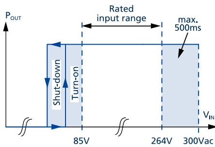
Fig. 3-1: Input voltage range
